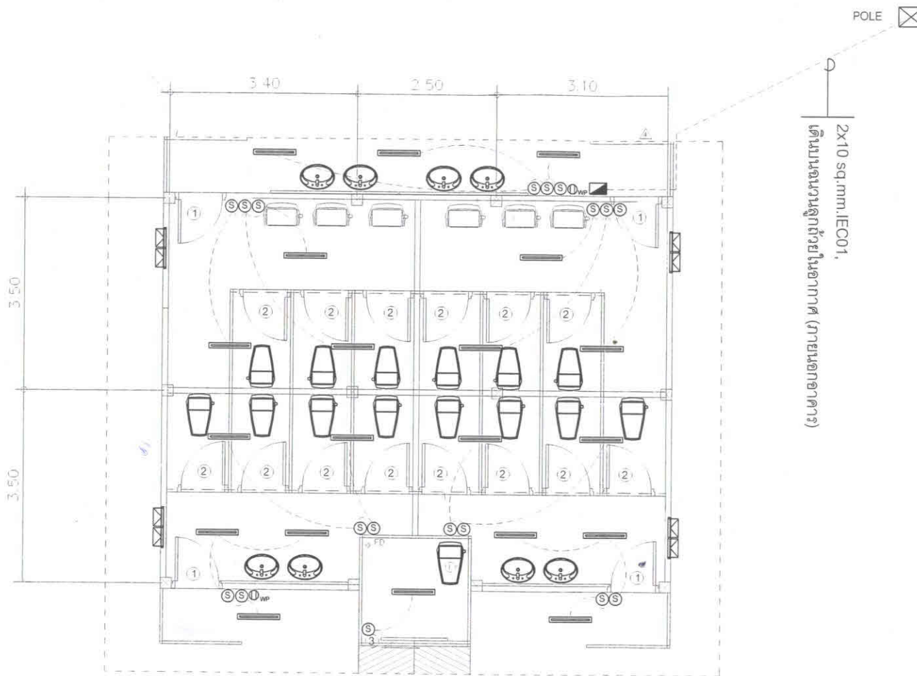
แปลนระบบไฟฟ้า มาตราส่วน 1:100
