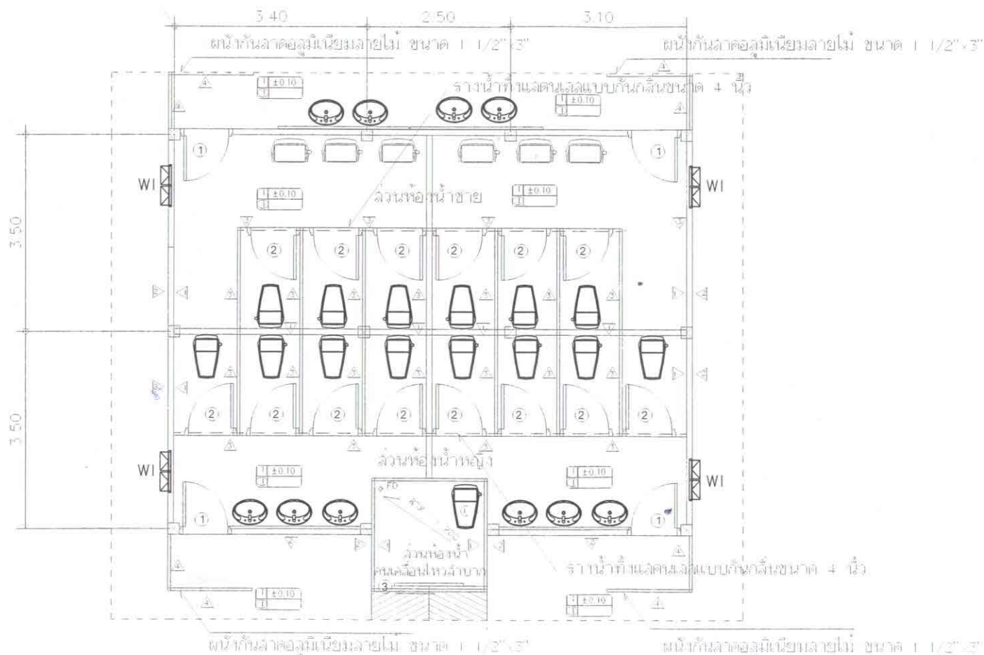
แปลนพื้นห้องน้ำ มาตรฐาน _____ 1:100
