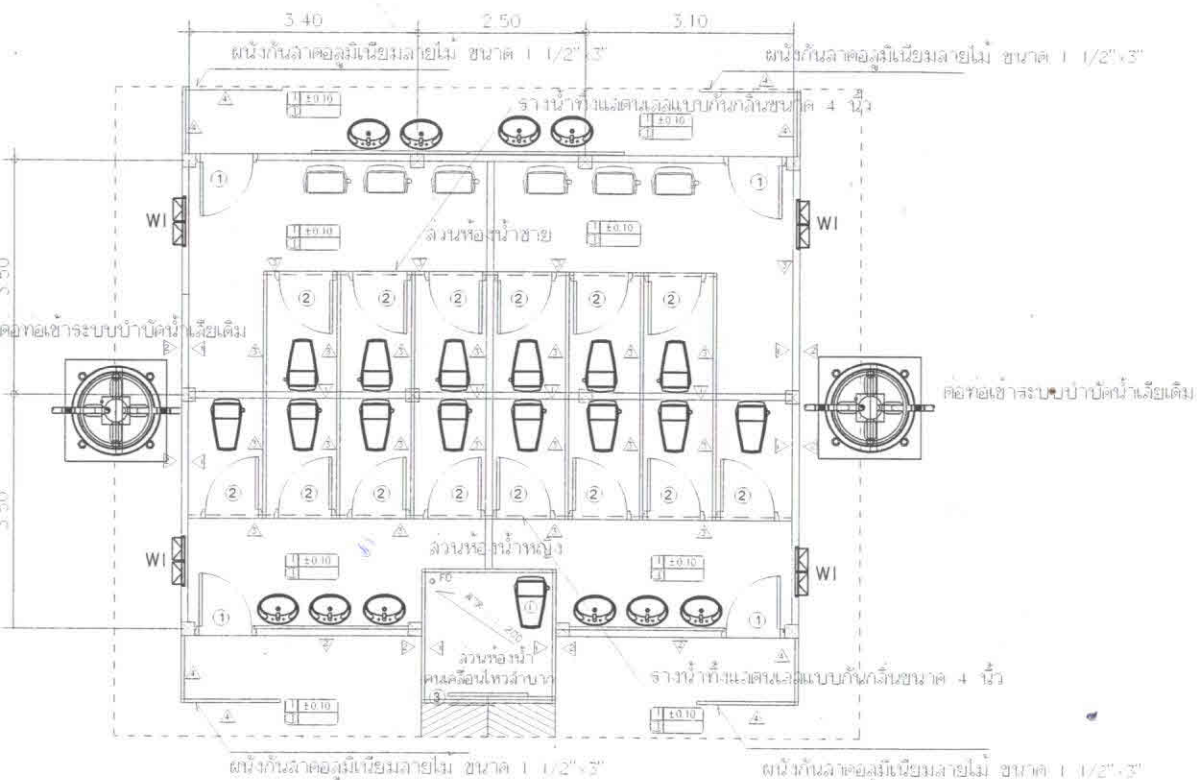
แปลนพื้นที่น้ำ มาตราส่วน 1:100
