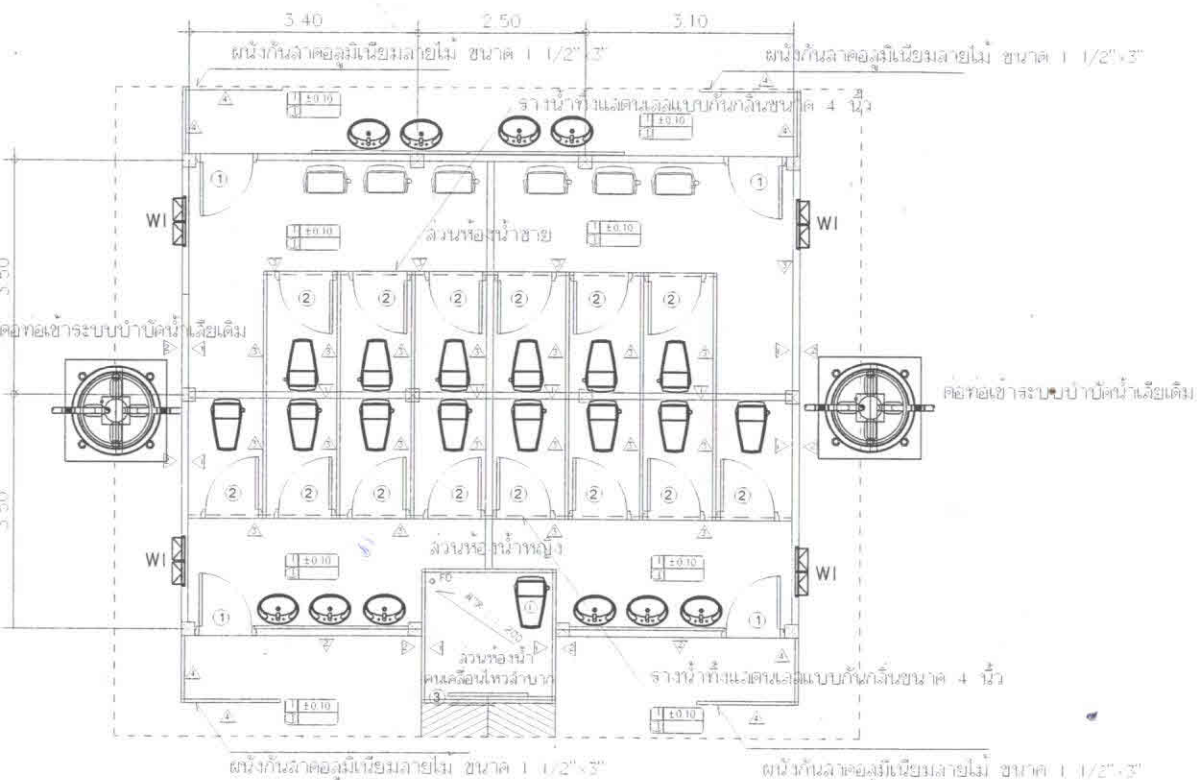
แปลนพื้นห้องน้ำ มาตราส่วน 1:100
