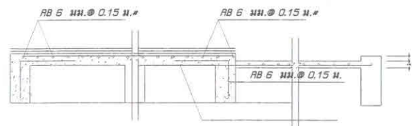
รูปขยายพื้นคอนกรีต มาตราส่วน 1:25
