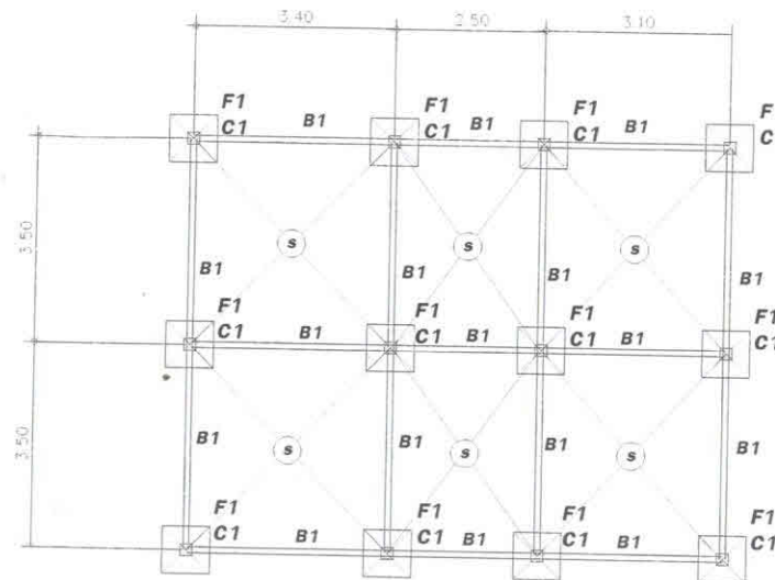
แปลนคาน คอดินและฐาน ราก มาตราส่วน 1:100
